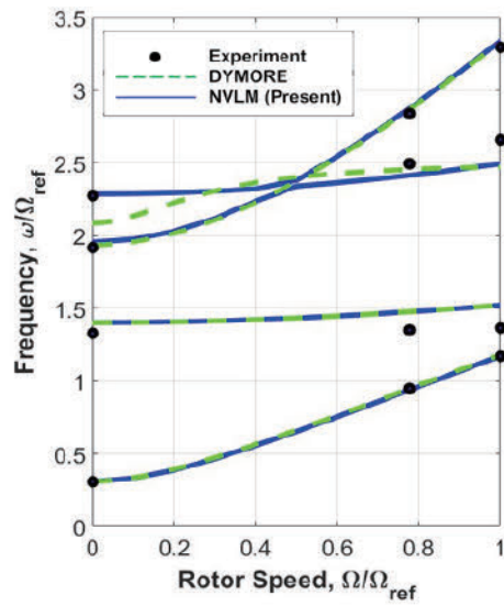
Fig. 8. Fan diagram
